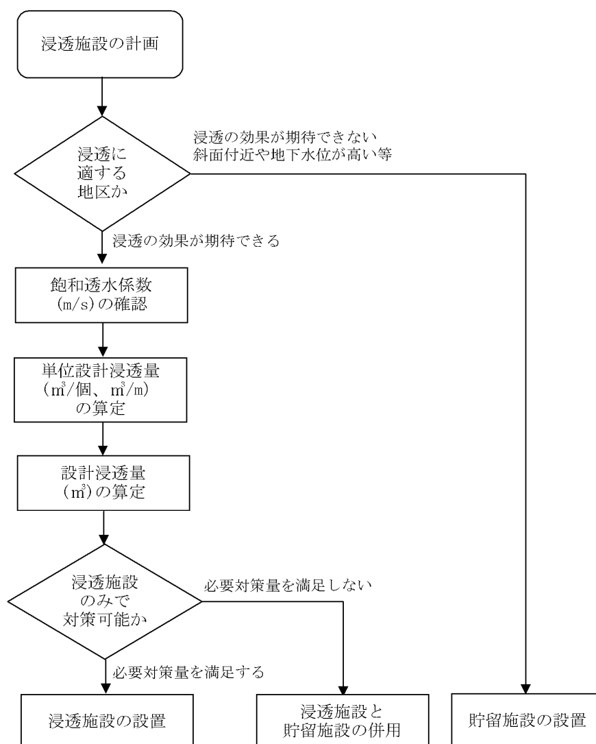
図 4 浸透施設の計画手順
