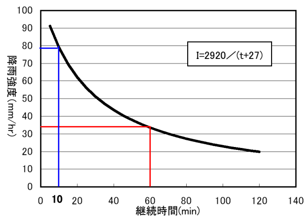
図 1 降雨強度式
